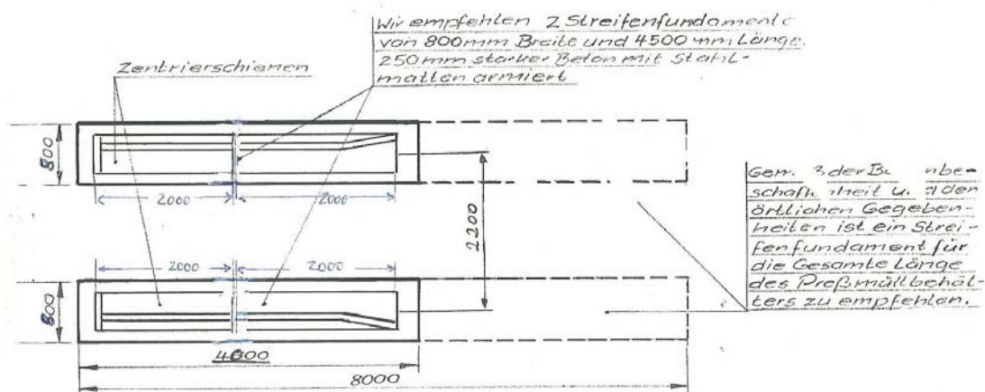
Zentrierschienen für RIES Sperrmüllpacker SP 320 für Abrollkipper
